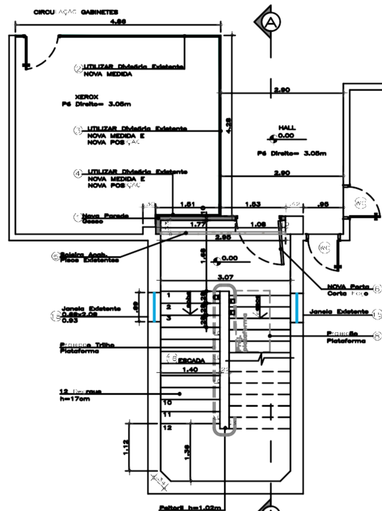
PLANTA ESCADA 3º ANDAR A CONSTRUIR
