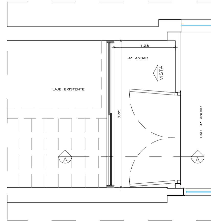
PLANTA JANELA
