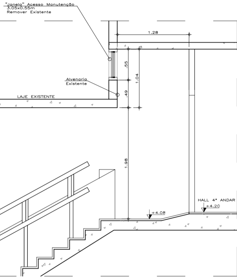
CORTE AA - JANELA
