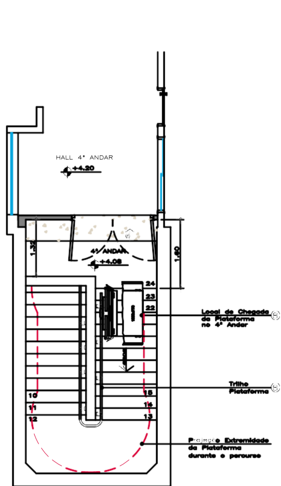
PLANTA ESCADA 4º ANDAR
