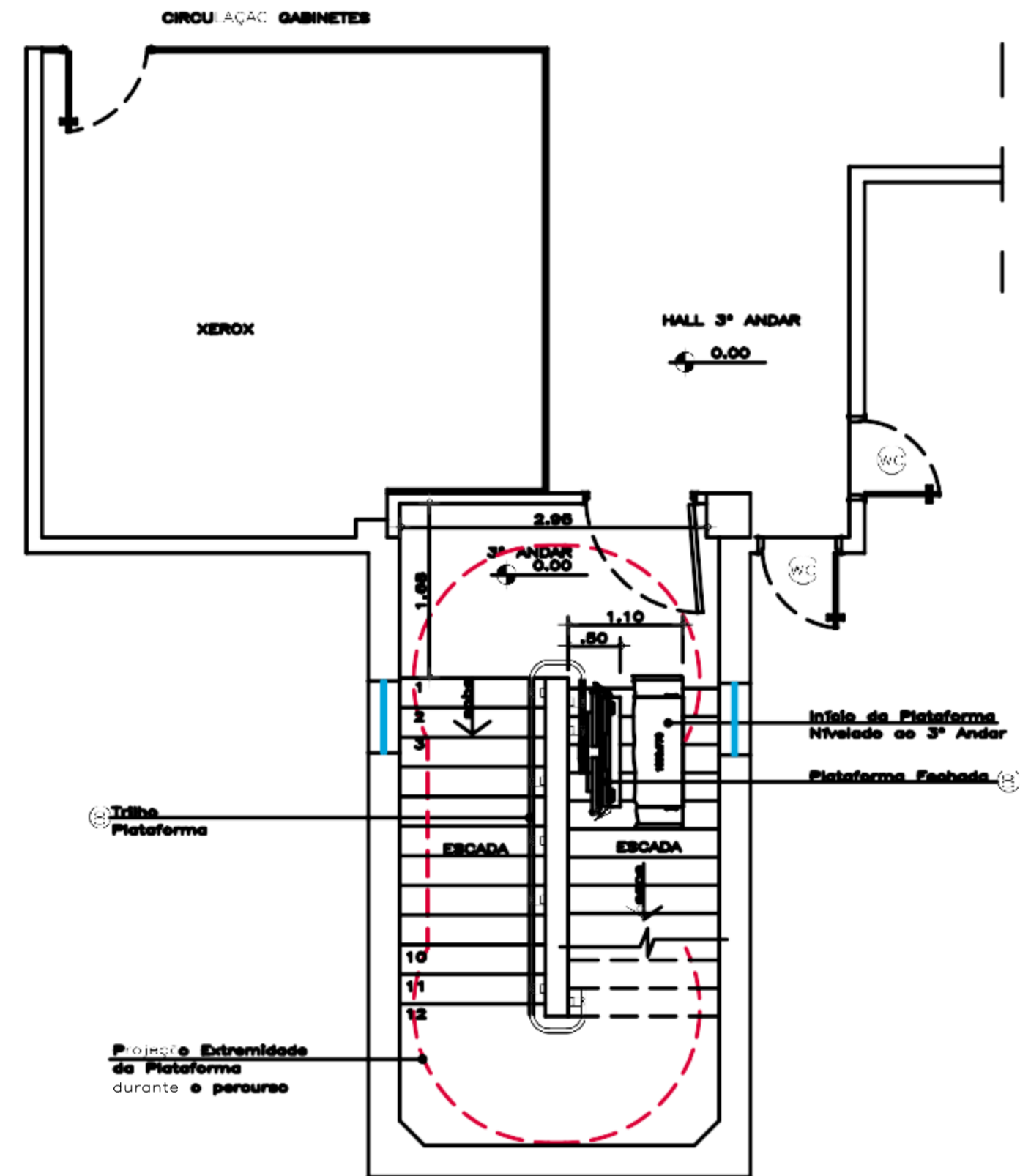
PLANTA ESCADA 3º ANDAR
